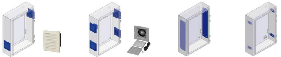
熱対策ルーバー 熱対策換気扇 側面鉄製基板 配線支持レール
