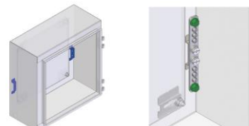
接地端子追加 増設アースバー
